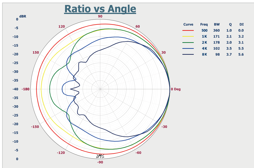
Круговая диграмма направленности громкоговорителя LPA-20K
